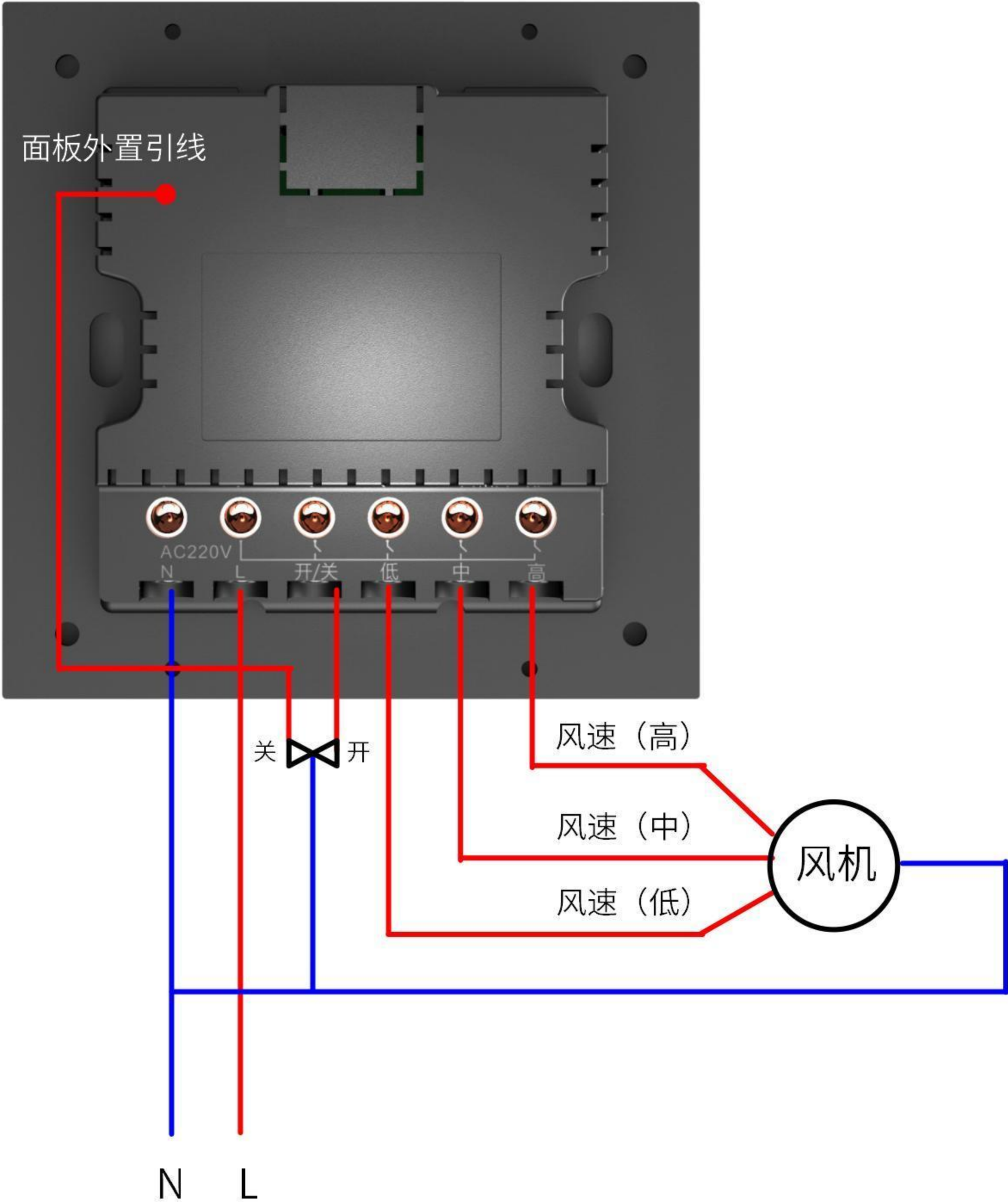
接线方法（二）
