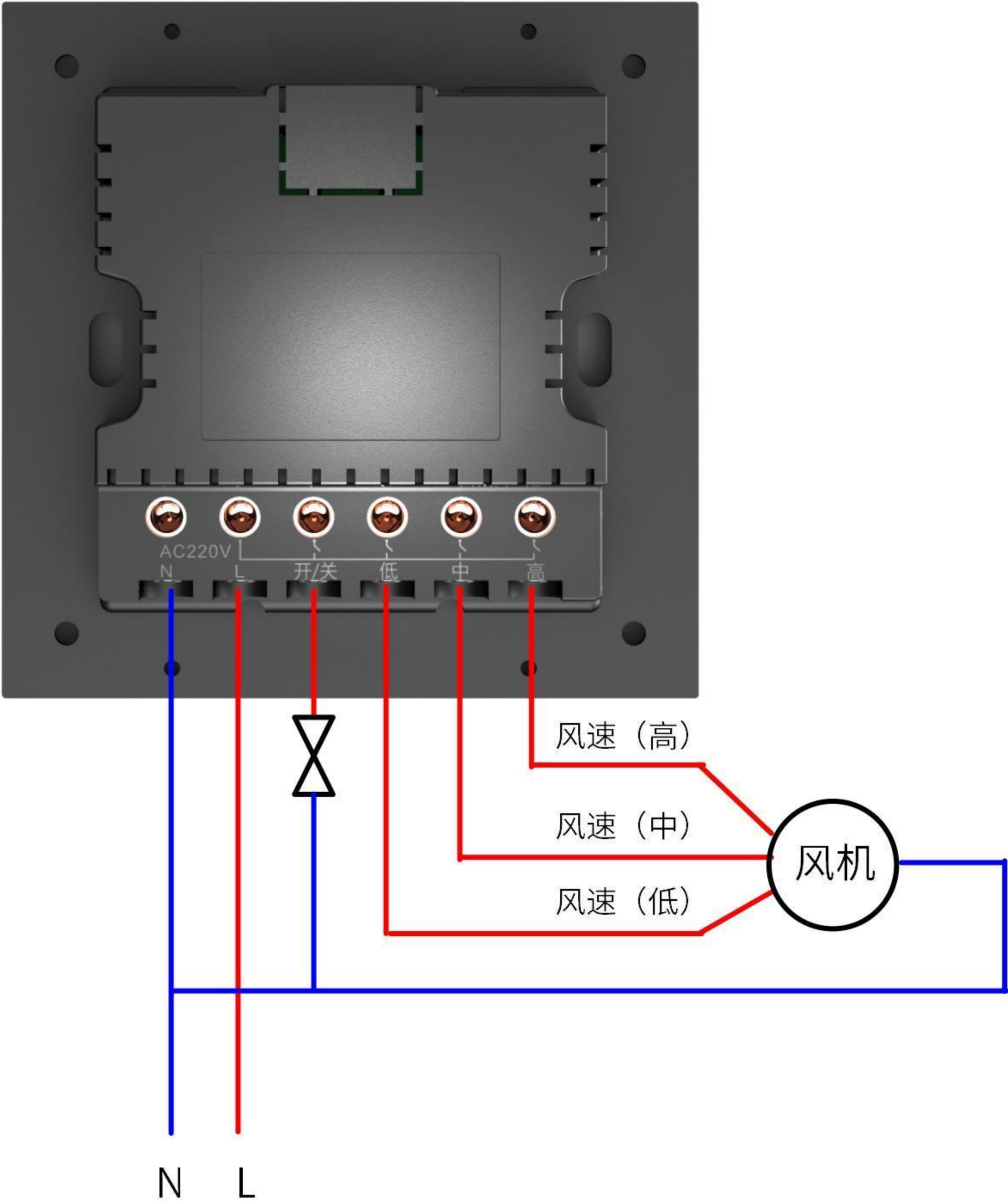
接线方法（一）
